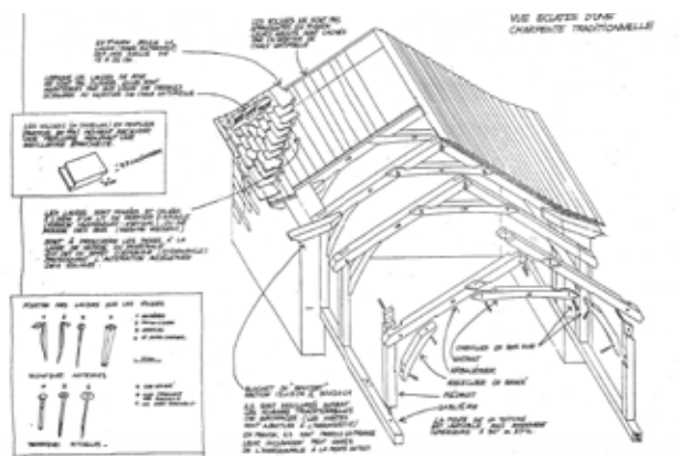
Illustration 35 : Détails d'une couverture en lauze
