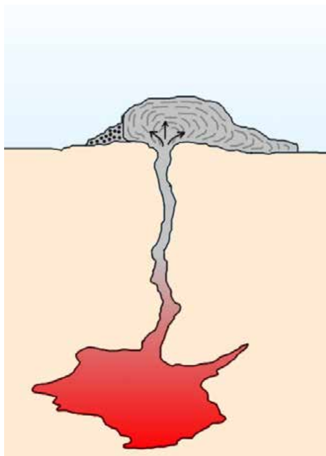
Illustration 18 : Formation d'un dôme-coulée - A. Aubry
